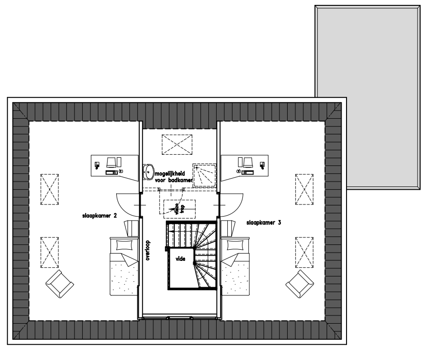
Verdiepingsvloer
