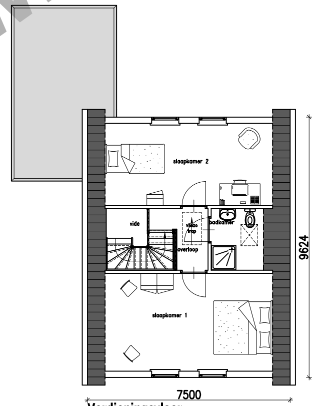
Verdiepingsvloer
