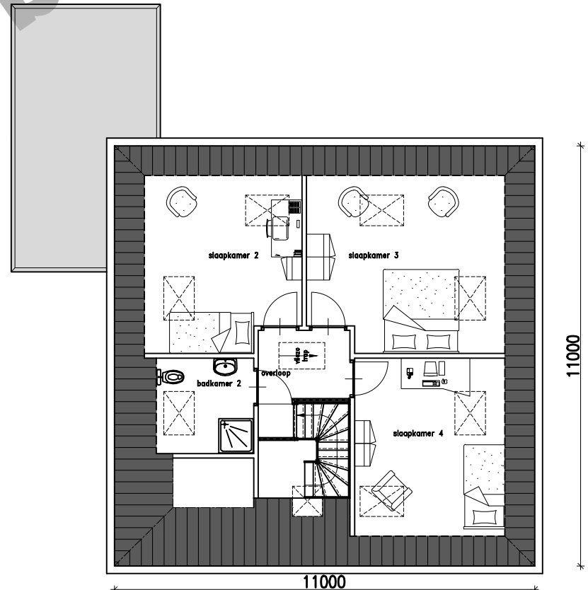
Verdiepingsvloer
